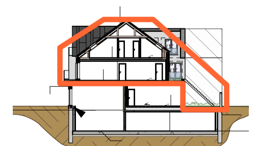
Doorsnede B-B
