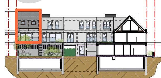
ACHTERGEVEL / DOORSNEDE A-A
